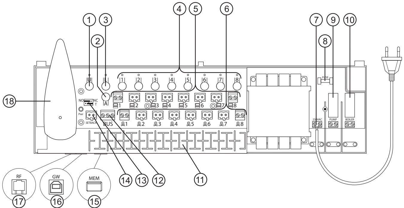
LK Mottagarenhet ICS-RF8.
