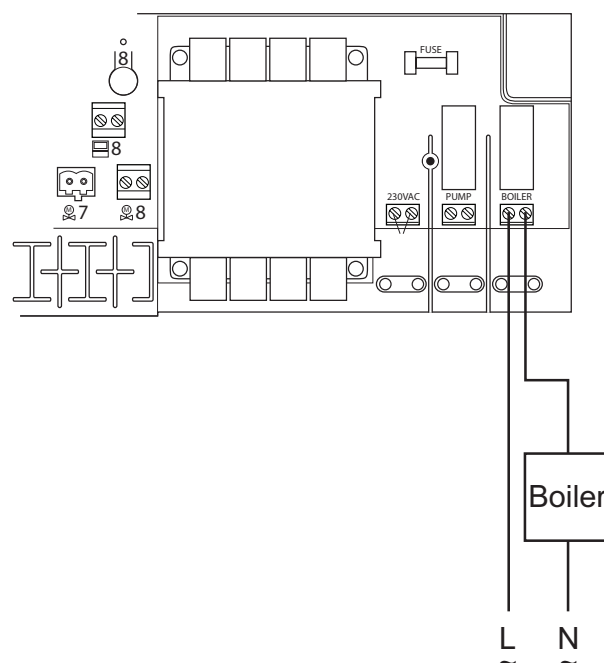
Kopplingschema för inkoppling av värmekälla till mottagarenhet ICS 8.
