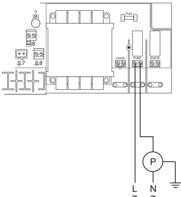
Kopplingschema för inkoppling av pump till mottagarenhet ICS 8.
